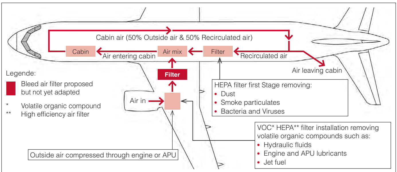
Schema für den Einsatz hocheffektiver Filter zur Vermeidung von Fume Events.
